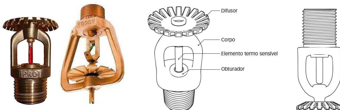
Figura 10 - Sistema Hidráulico (Chuveiros automáticos). Fonte: DSCI- CBPMESP
